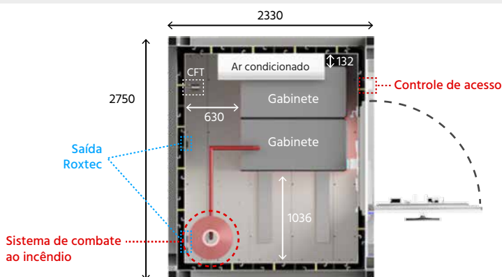
Layout Rack seguro para 2 gabinetes - içável
